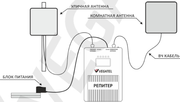
СХЕМА ПОДКЛЮЧЕНИЯ РЕПИТЕРА
